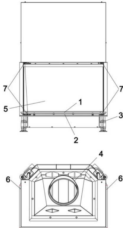
Abb. 1: Bauteile der Panorama-Kamine (schematisch)
